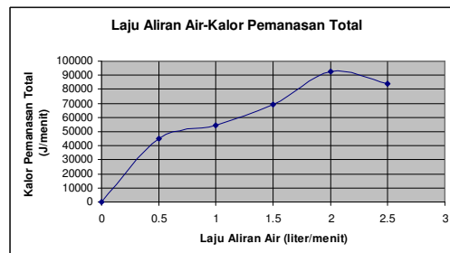
Gambar 8 Hubungan Laju Aliran Air dengan Kalor Pemanasan Total.
