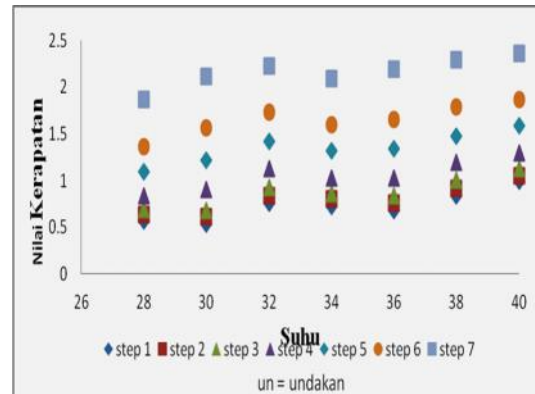
Gambar 1. Grafik hubungan antara suhu cairan pengembang dengan nilai kerapatan
