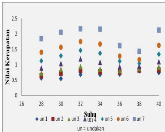
Gambar 2. Grafik hubungan antara suhu cairan fixer dengan nilai kerapatan.
